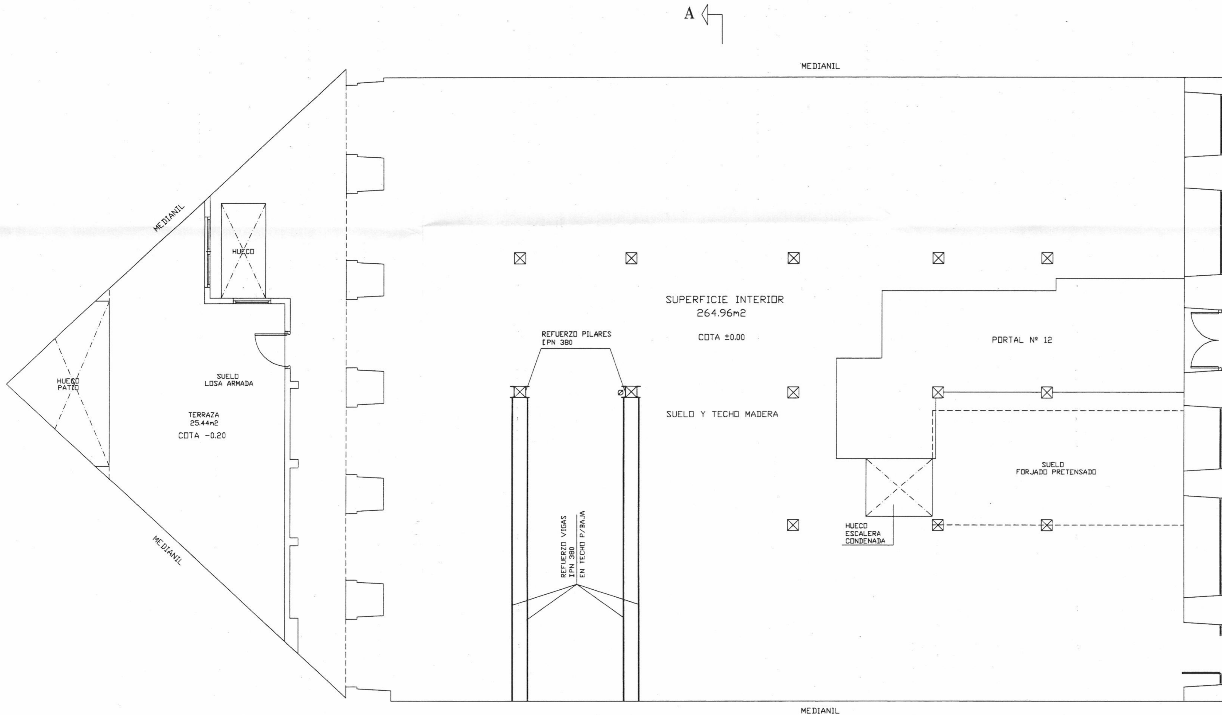
PLANTA BAJA
