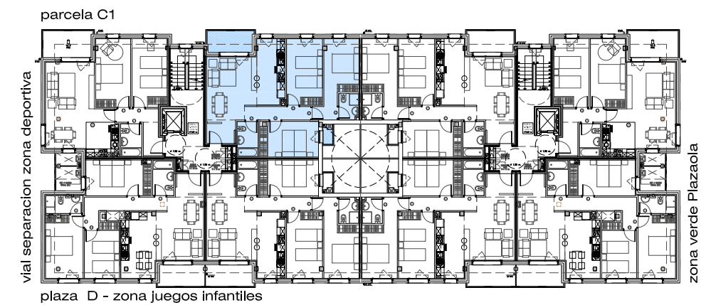
localizacion de la vivienda en planta
